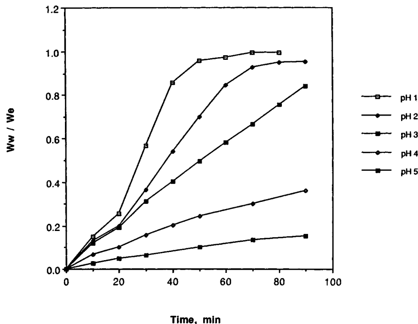
Figure 5 Swelling pH dependency; 78/22 mol % HEMA/DMA gel; formic acid buffer. (—□—) pH 1; (—◆—) pH 2; (—□—) pH 3; (—◇—) pH 4; (—■—) pH 5.
