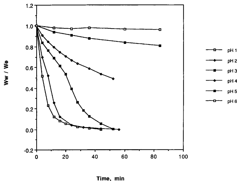
Figure 9 Deswelling pH dependency; 78/22 mol % HEMA/MAA gel; formic acid buffer. (—□—) pH 1; (—◆—) pH 2; (—□—) pH 3; (—◇—) pH 4; (—■—) pH 5; (—□—) pH 6.
