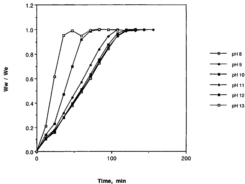
Figure 4 Swelling pH dependency; 78/22 mol % HEMA/MAA gel; (—□—) Imidazole buffer, pH 8; (—◆—) pH 9; (—□—) pH 10; (—◇—) pH 11; (—■—) pH 12; (—□—) pH 13.
